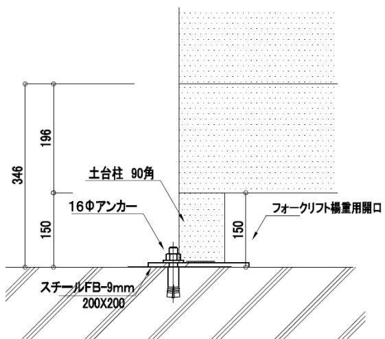
土台部詳細図
