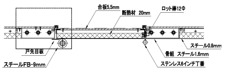
平面詳細図
