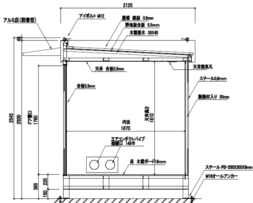
断面図
