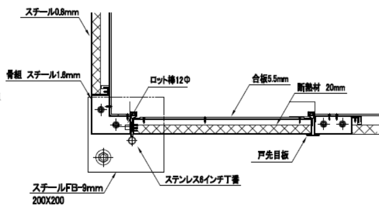
平面詳細図
