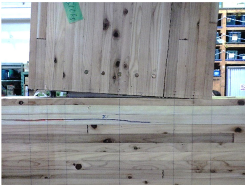
ビスの位置でのひび割れ
