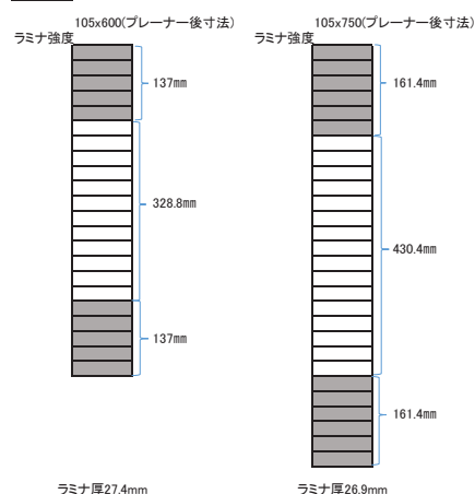
ヒノキ集成材ラミナ構成
