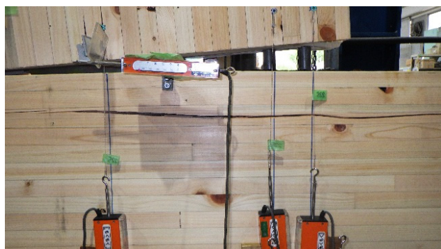
パネルゾーン割裂破壊
