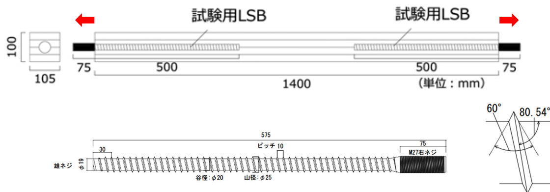
接合具：ラグスクリーボルト (LSB) φ 25
