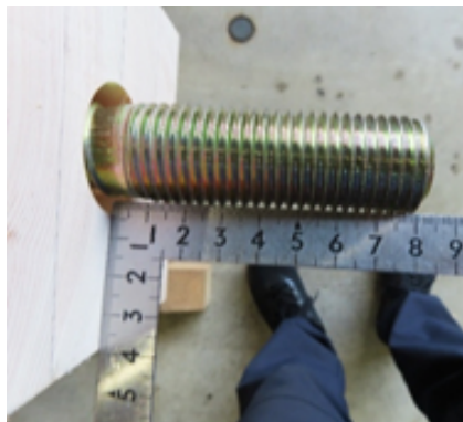
写真 1 LSB 引き抜け
