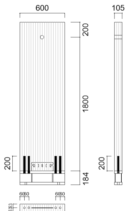
試験体図（単位：mm）
