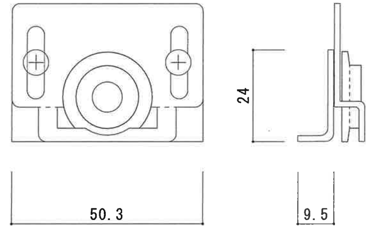
K J 108S F型戸車
