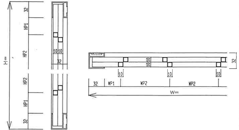
断面図
