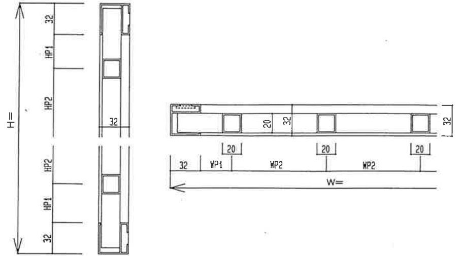
断面図
